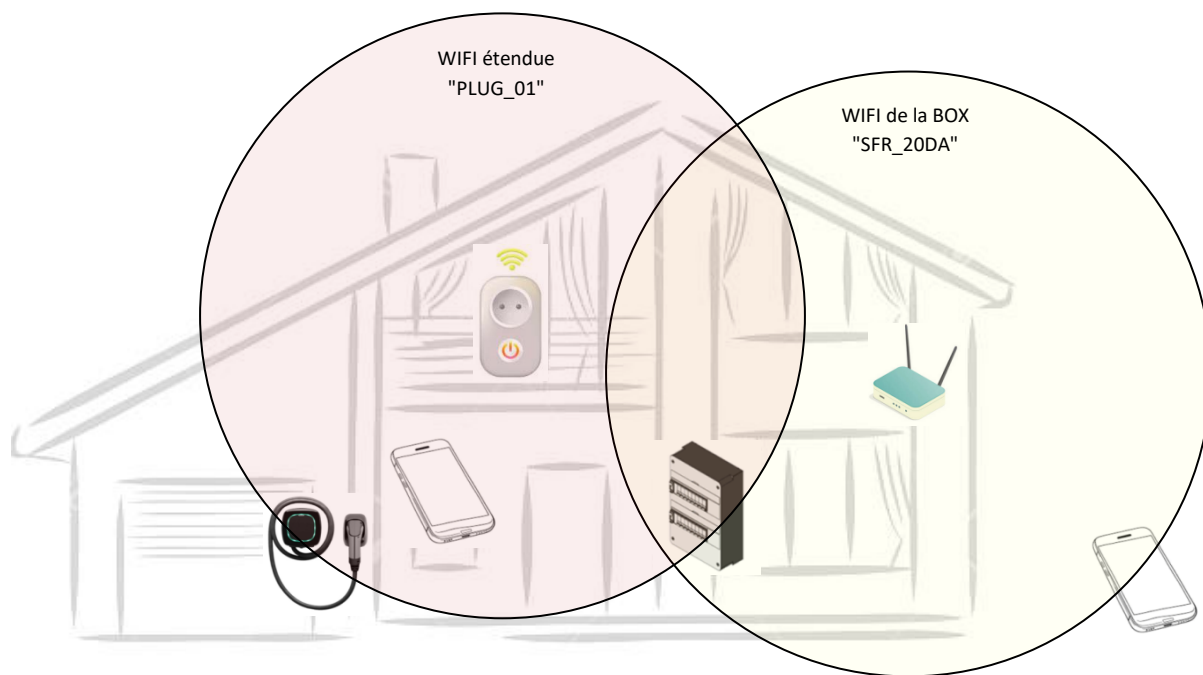
Figure 8 : SmartCharger intégré dans la couverture WIFI étendue "PLUG_01" et le Module TIC sur la couverture WIFI de la BOX "SFR_20DA" sur le même LAN
