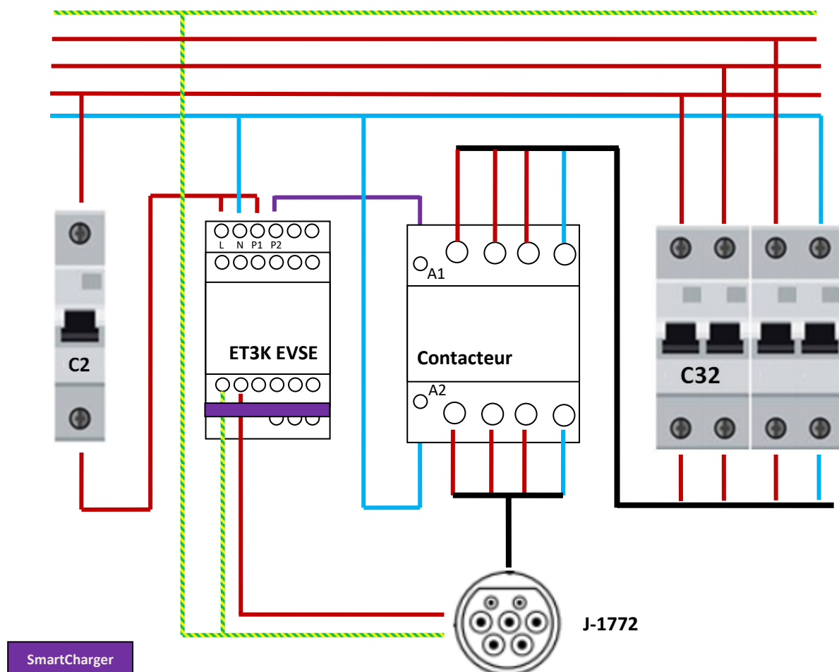
Figure 3 : Schéma de câblage de l'ET3K en 400 V Triphasés
