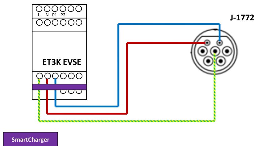
Figure 5 : Câblage du Proximity Pilot en mode Socket
