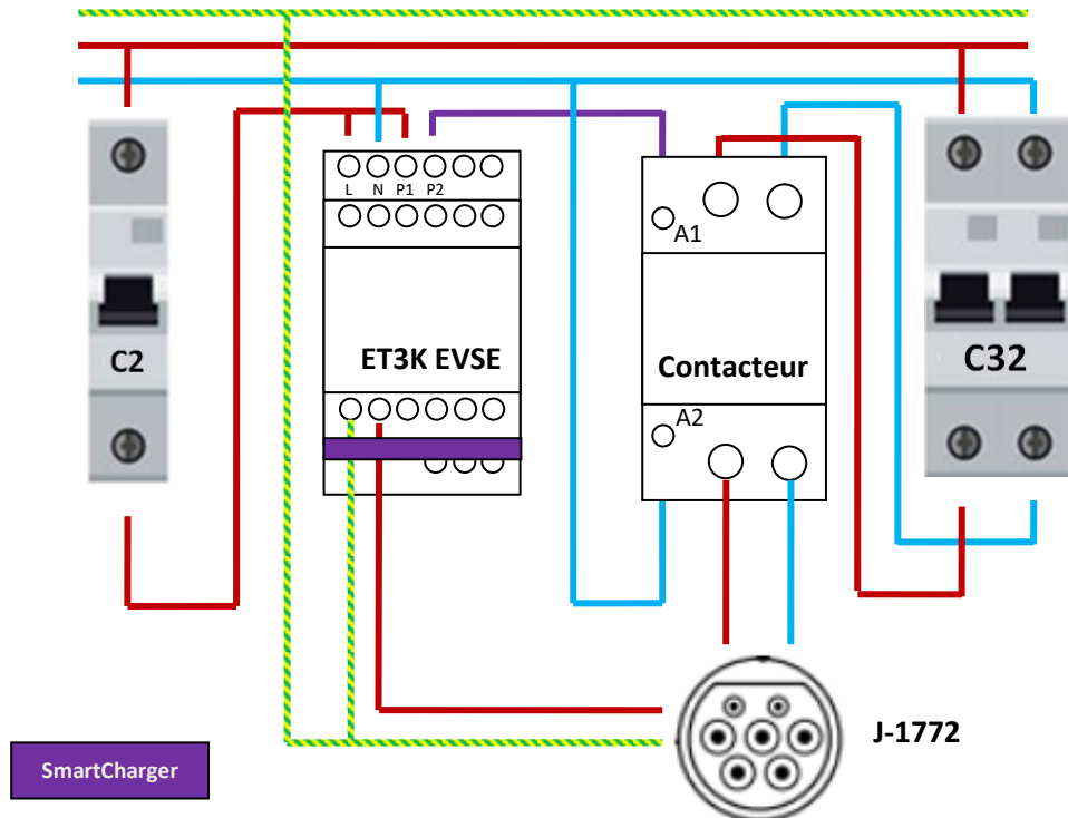
Figure 2 : Schéma de câblage de l'ET3K en 240 V Monophasé
